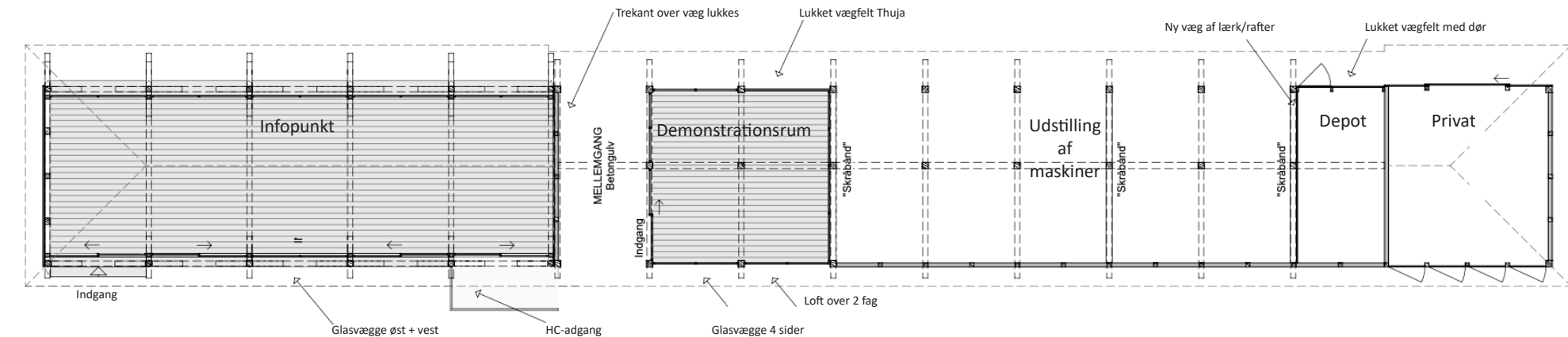
Planskitse af Infocenteret v/Arkitektfirma Mette Maegaard Nielsen APS.
